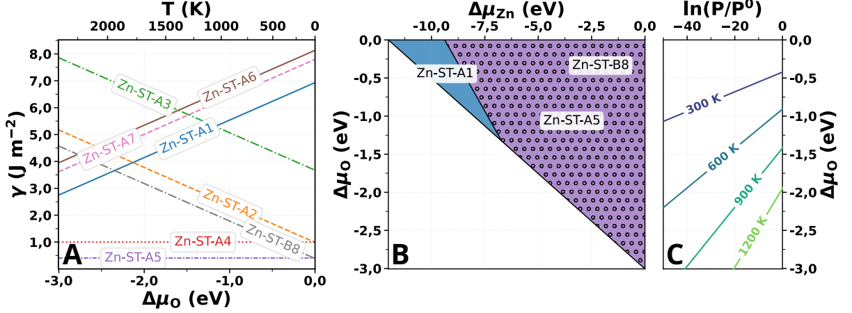
Figura 9: (A) \gamma em função de \Delta\mu_O para as diferentes terminações superficiais (010) do ZnWO_4 (B) Diagrama de estabilidade das terminações superficiais (010) em função de \Delta\mu_O e \Delta\mu_{Zn} . (C) Relação de T para diferentes \Delta\mu_O e pressões parciais de O_2 .
