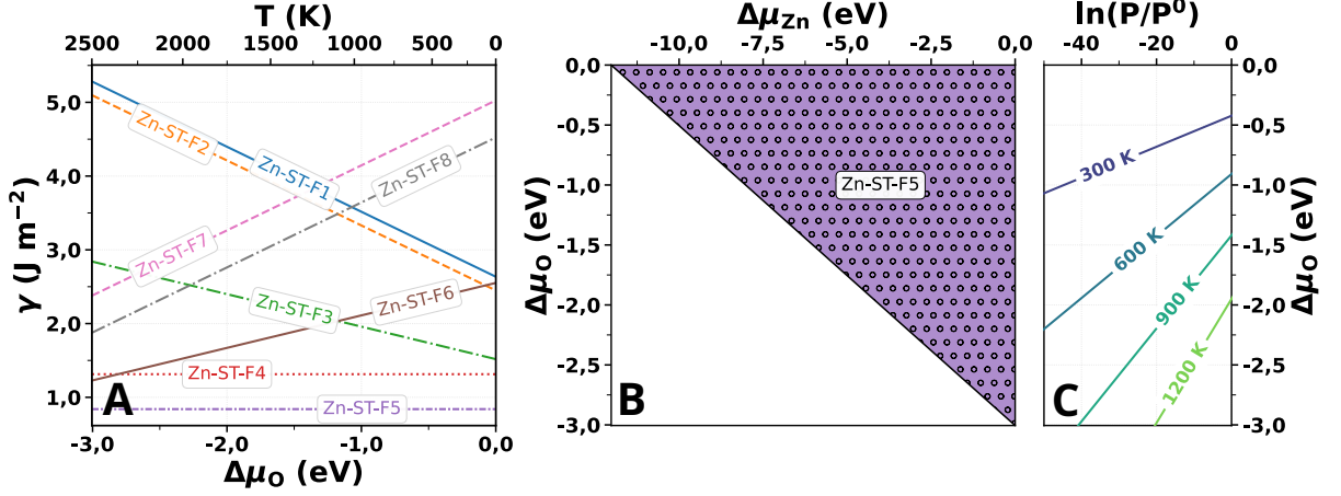
Figura 16: (A) \gamma em função de \Delta\mu_O para as diferentes terminações superficiais (110) do ZnWO_4 (B) Diagrama de estabilidade das terminações superficiais (110) em função de \Delta\mu_O e \Delta\mu_{Zn} . (C) Relação de T para diferentes \Delta\mu_O e pressões parciais de O_2 .
